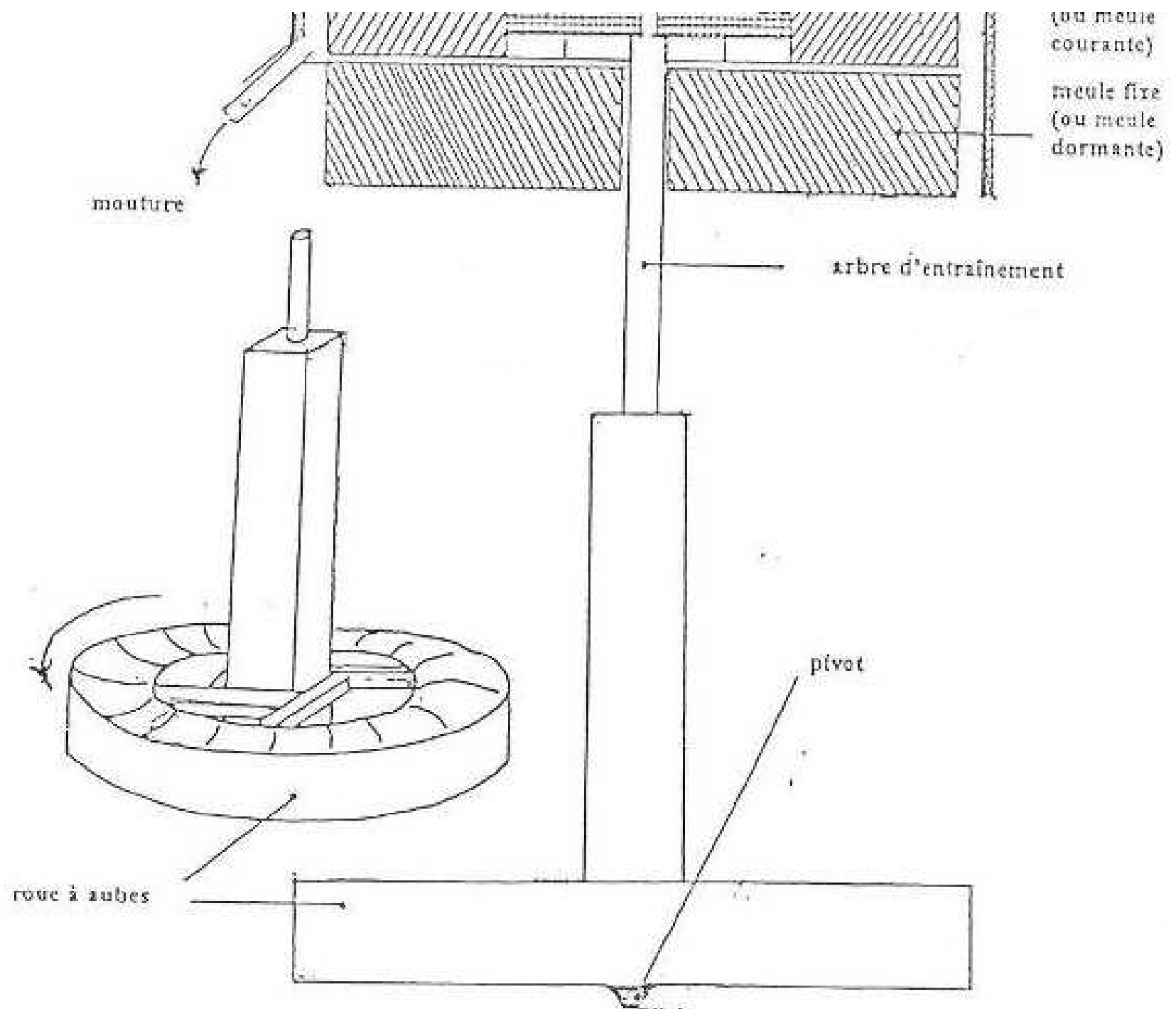
Croquis de la mairie de Sazos, pour la visite des moulins
