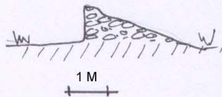
COUPE AA
