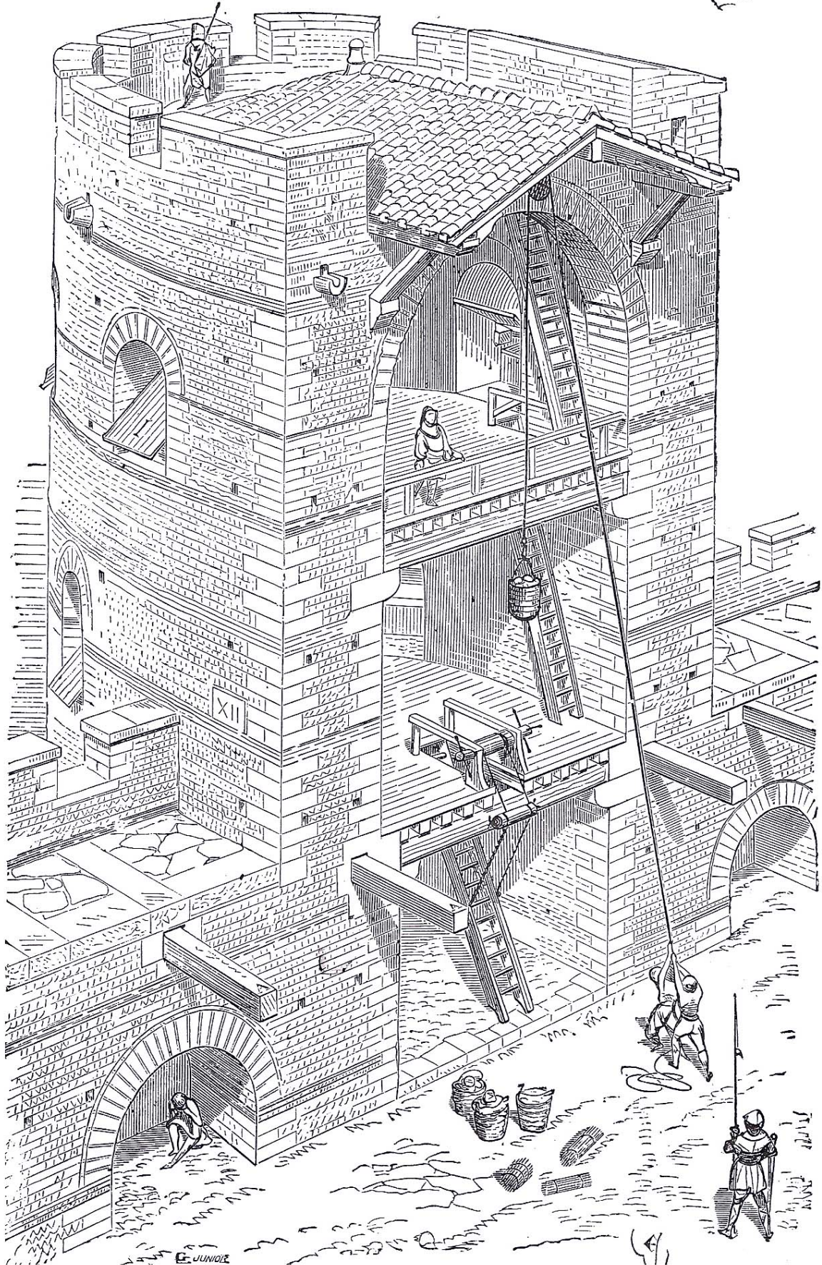
MODELE DE TOUR A GORGE OUVERTE DESSIN DE VIOLET LE DUC ENCYCLOPEDIE MEDIEVALE INTERLIVRES
