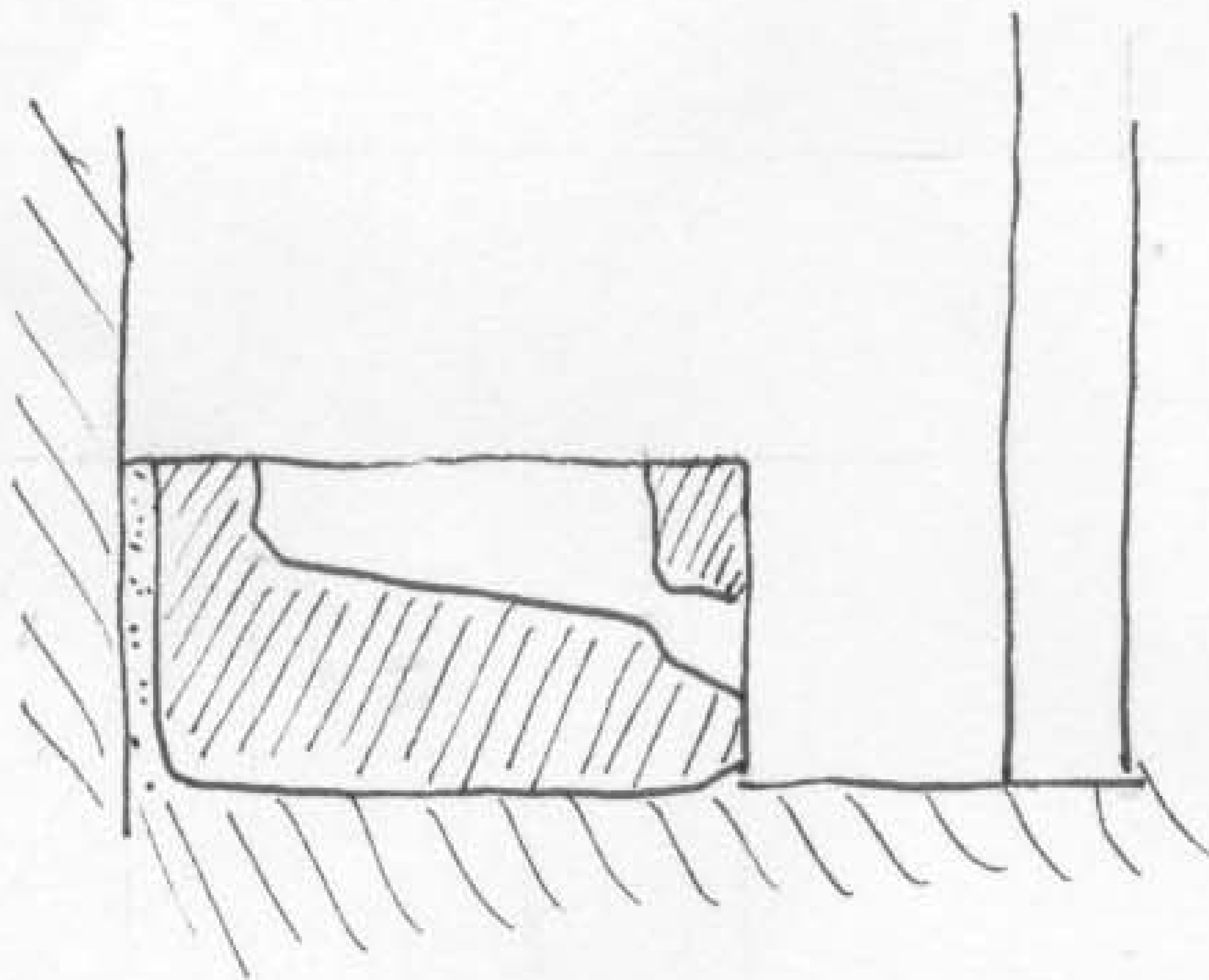
COUPE AA
