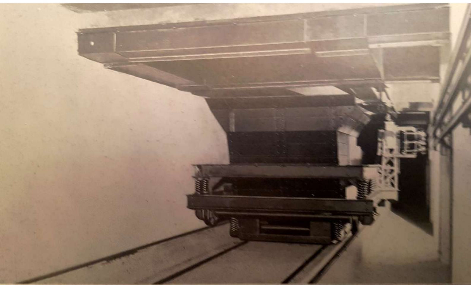
FIG. 5. — Wagonnet de décrochage.
