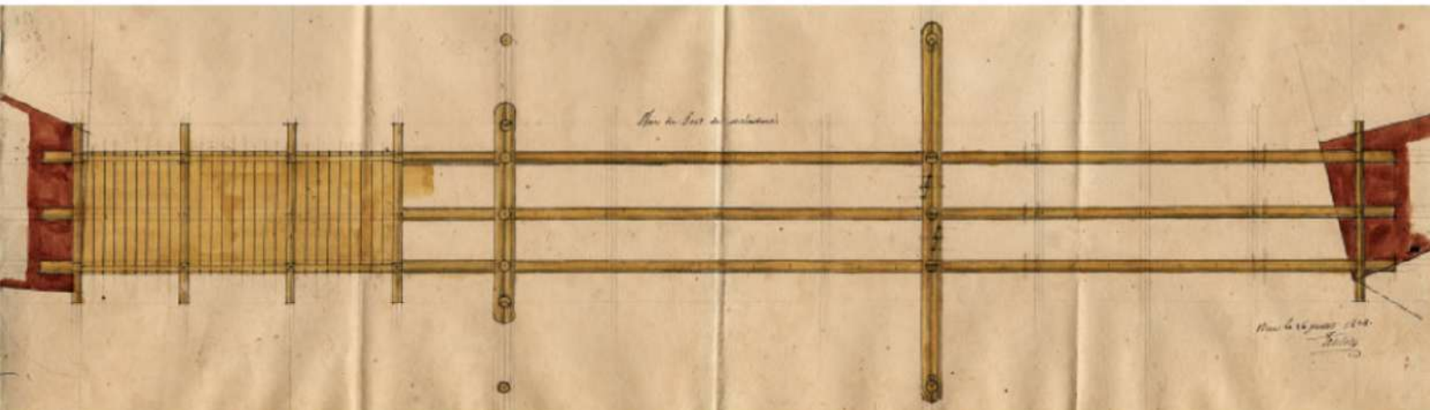
Pont de Malaussène, élévation et plan, 26 juillet 1808. Archives départementales des Alpes-Maritimes, CE S 49.
