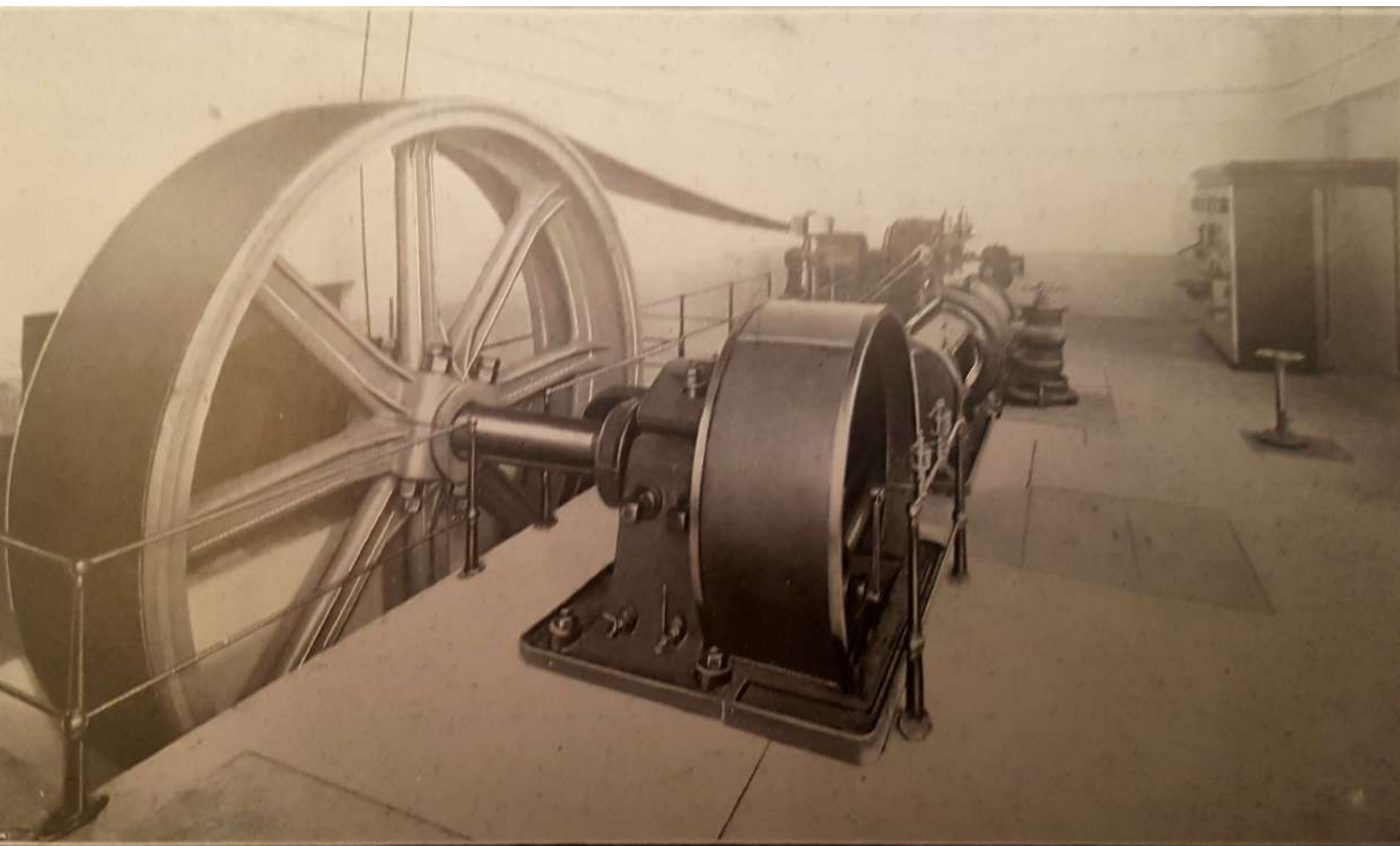
FIG. 6. — Machine à vapeur et alternateur.
